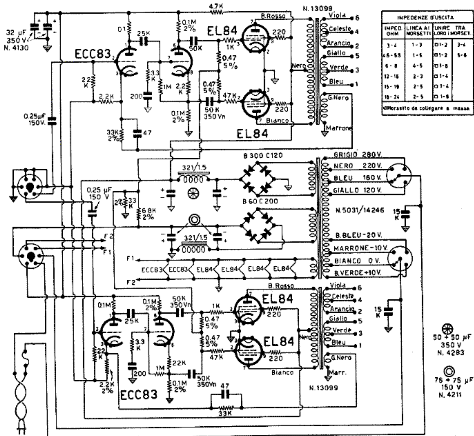
AMPLIFICATORE STEREO G.236
